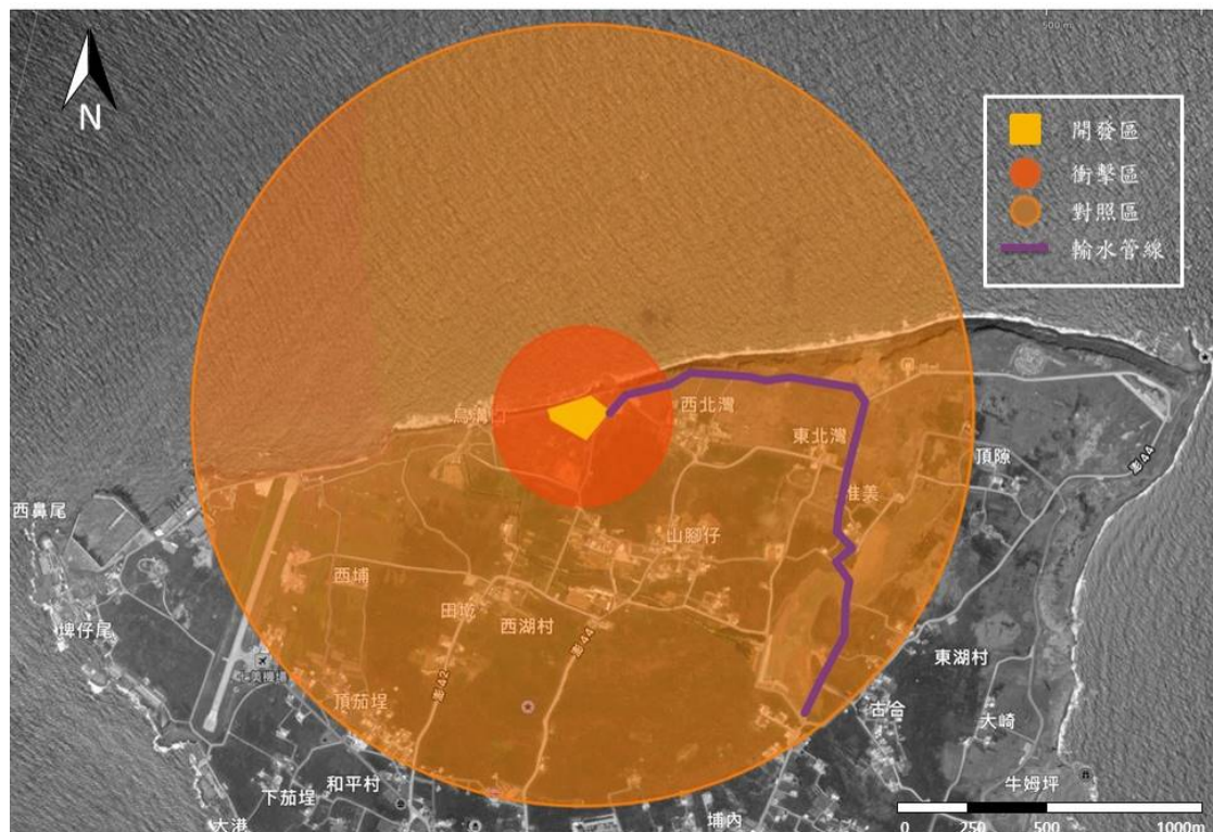
輸水管線
