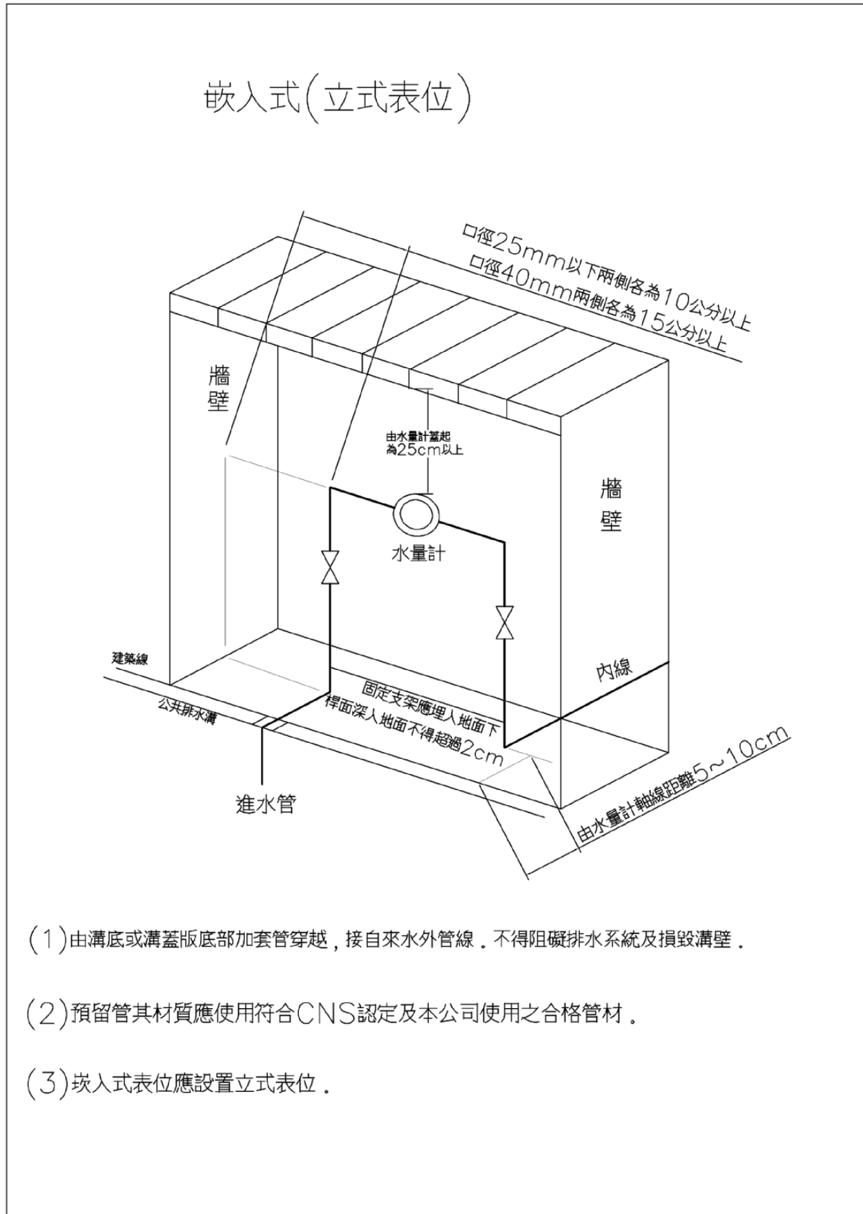
參考圖例 2-1：嵌入式表位空間
