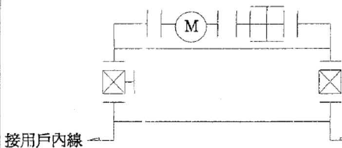
Ø 50mm~100mm 立式表位按裝組合參考示意圖
