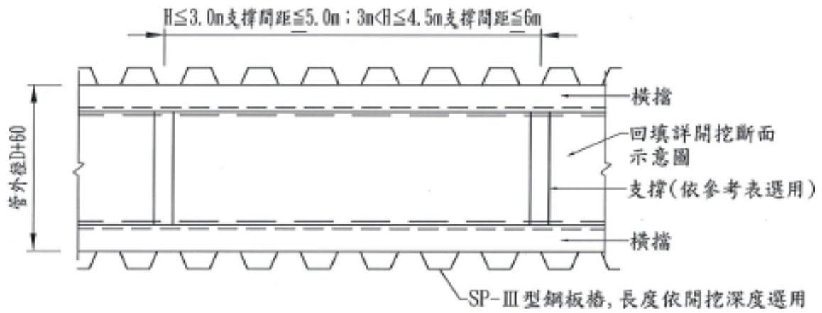
圖 3-5 鋼板樁擋土設施平面圖
