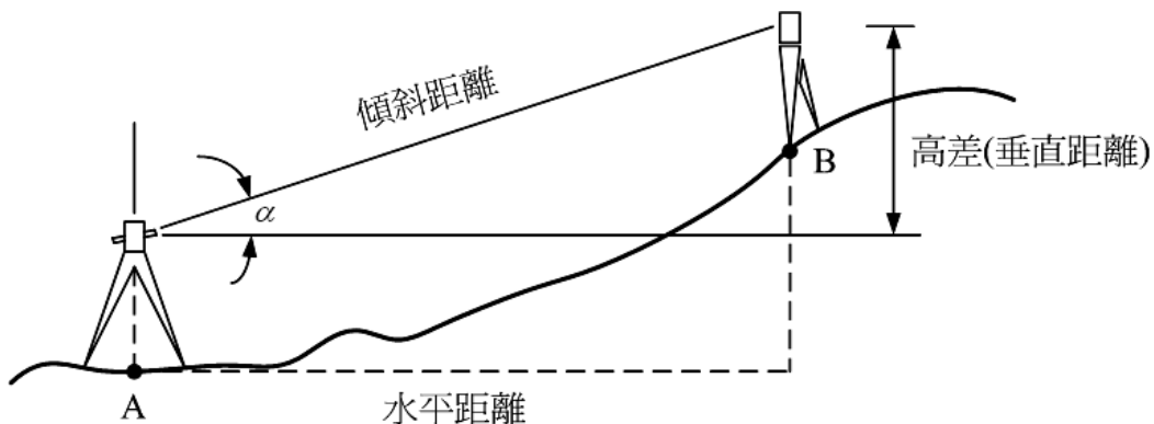
圖 6- 1 電子測距儀測距原理
