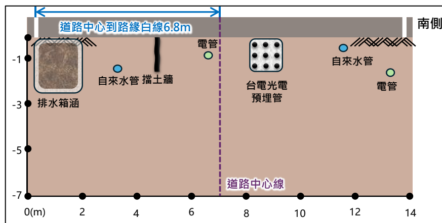
圖 2- 2 地下管線探挖斷面示意圖
