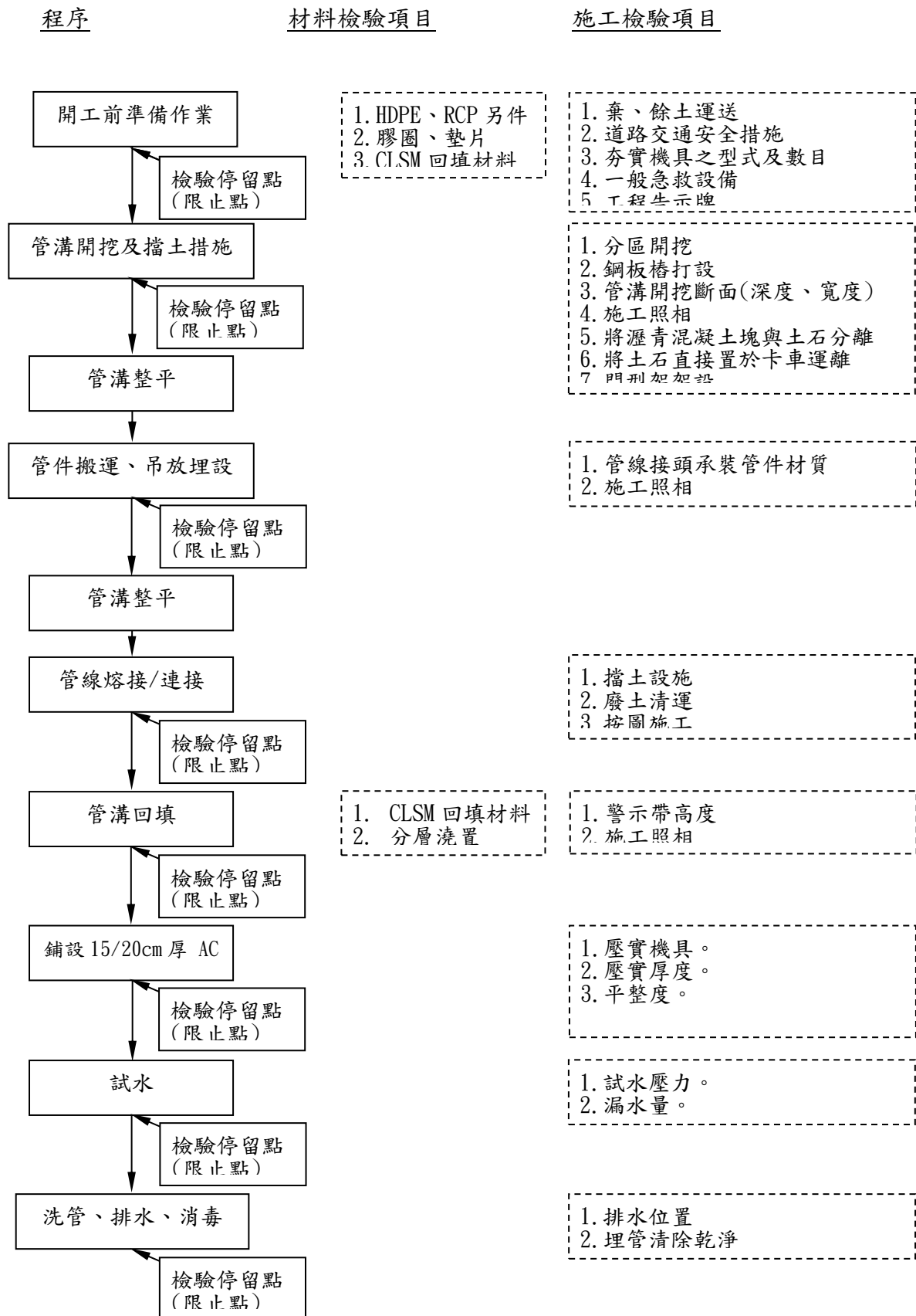
圖 3- 7 施工檢驗程序圖
