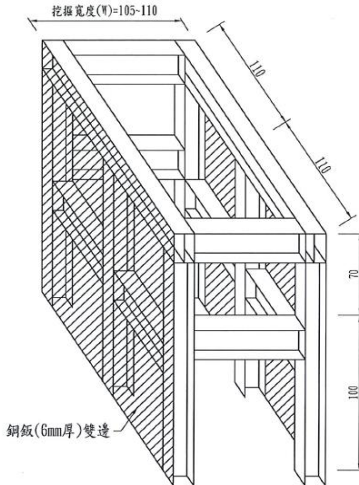
圖 3-6 門型框架擋土設施示意圖
