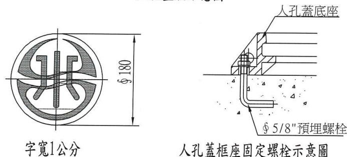
人孔蓋版示意圖
