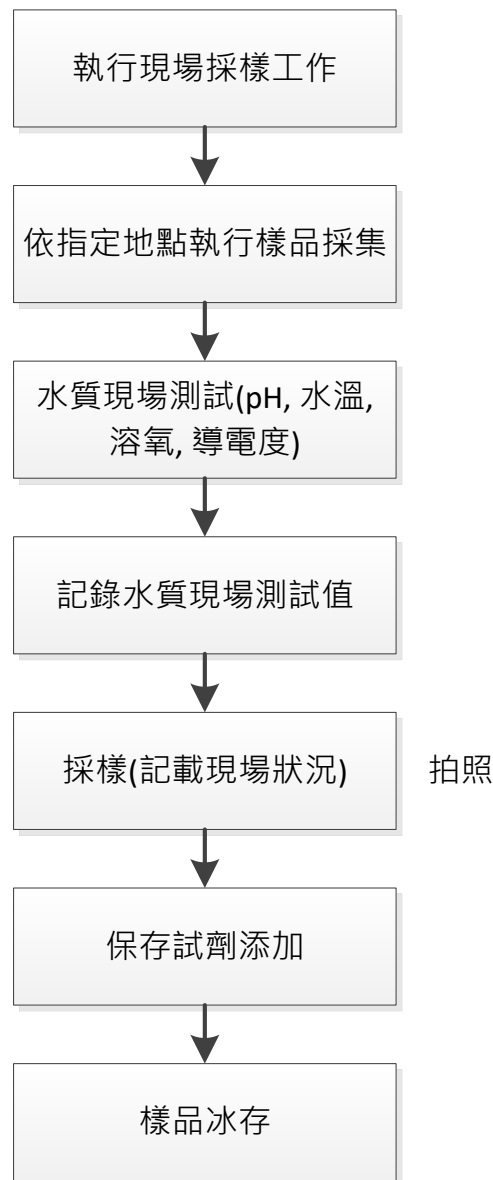
圖 1.5-5 地面水質現場監測作業流程圖
