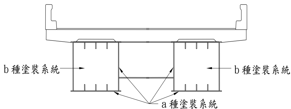
圖二、鋼箱型梁橋塗裝示意
