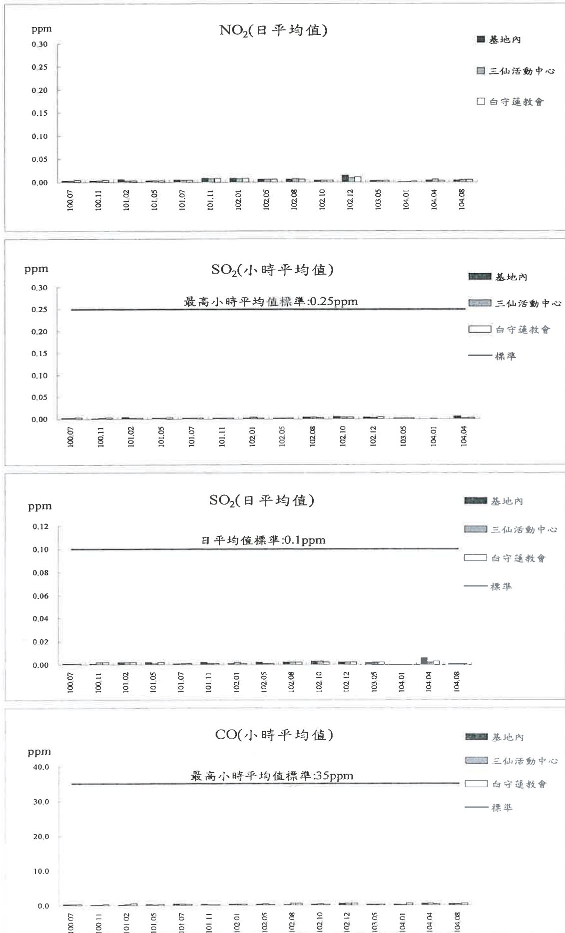
圖3.1-1 歷次空氣品質測值變化圖(續一)
