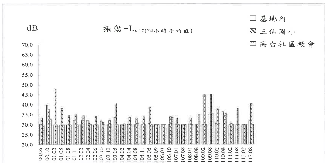
圖3.3-1 歷次振動測值變化圖
