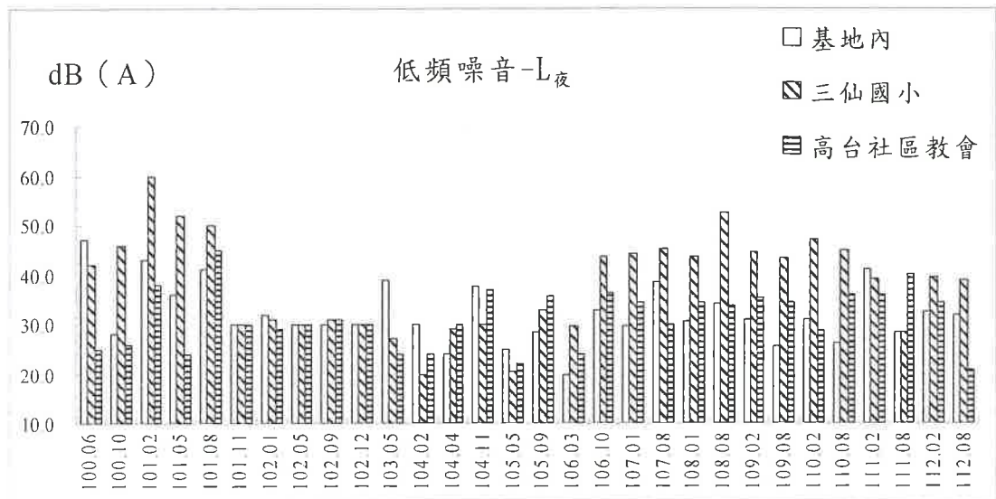
圖3.4-1 歷次低頻噪音測值變化圖
