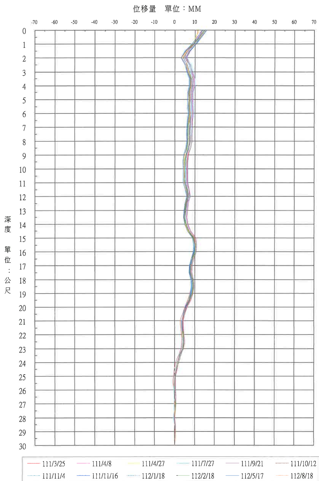
圖2.8-2 傾斜管測量位量曲線圖(SI1-B)
