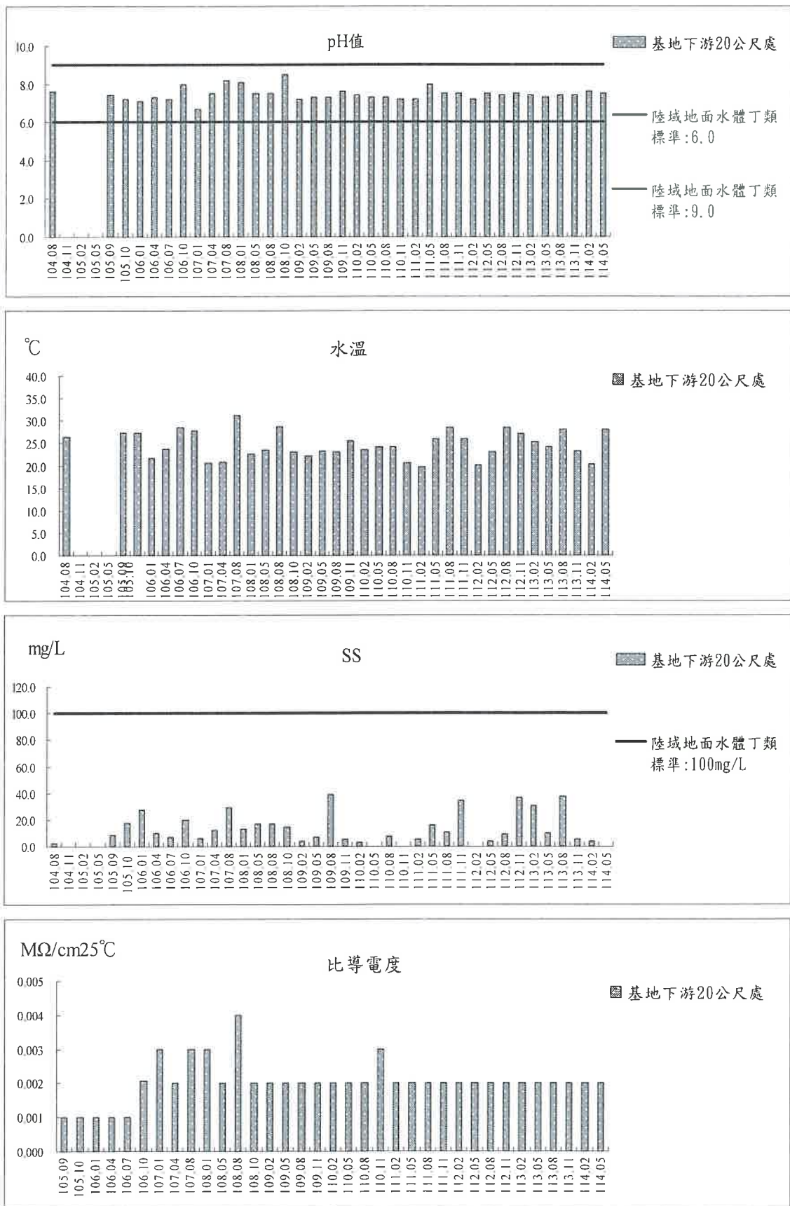
圖 3.5-2 基地下游 20 公尺處地面水水質監測結果趨勢圖
