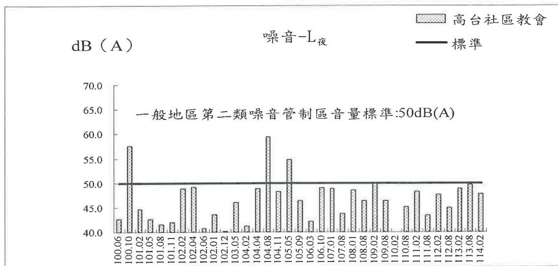
圖3.2-3 高台社區教會歷次噪音測值變化圖
