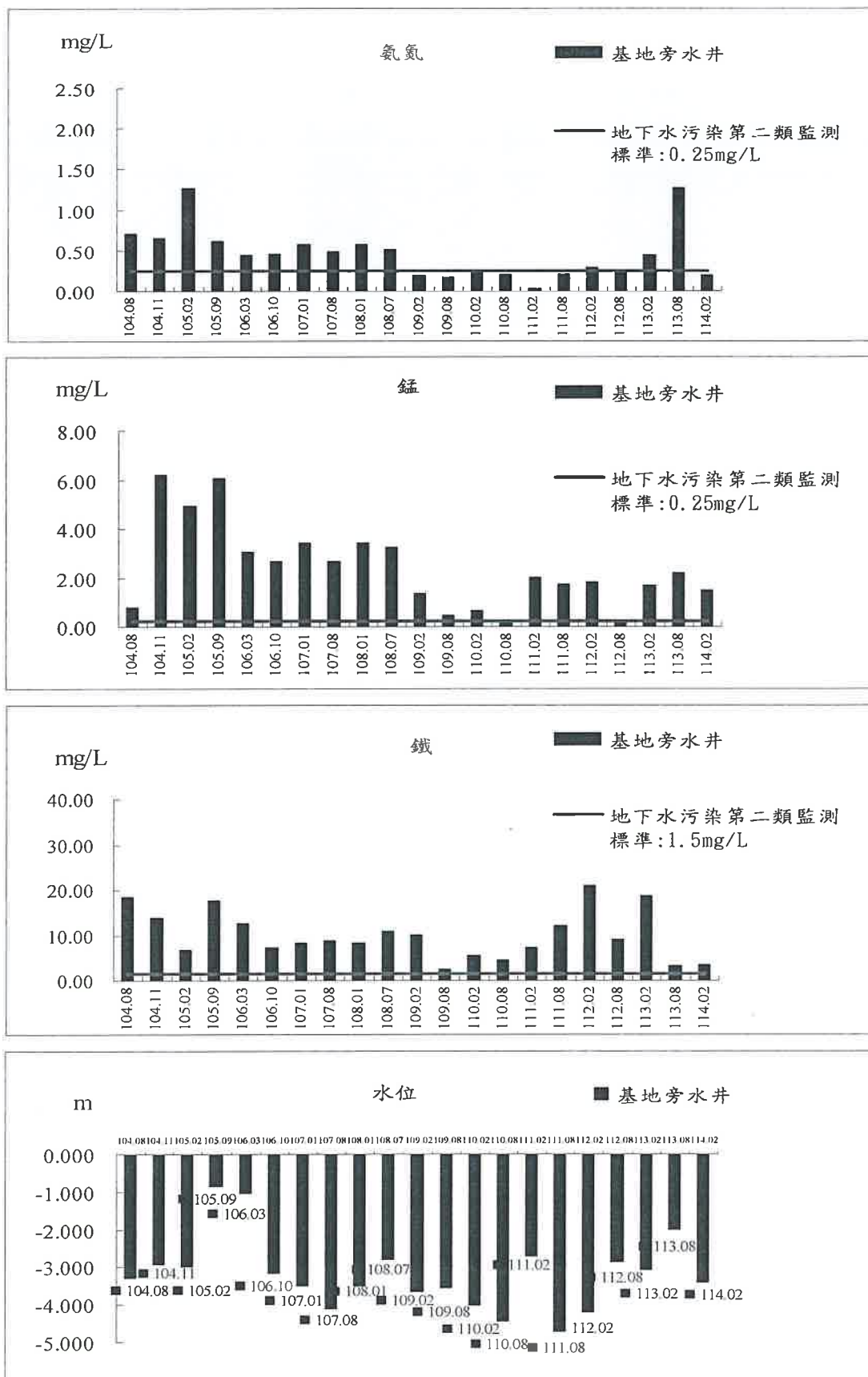
圖 3.7-1 地下水水質監測結果趨勢圖
