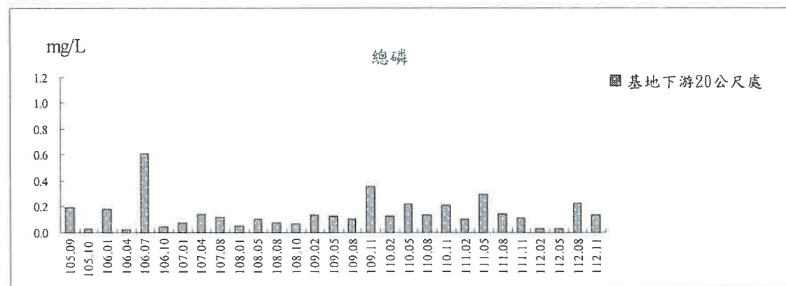
圖 3.5-2 基地下游 20 公尺處地面水水質監測結果趨勢圖(續一)
