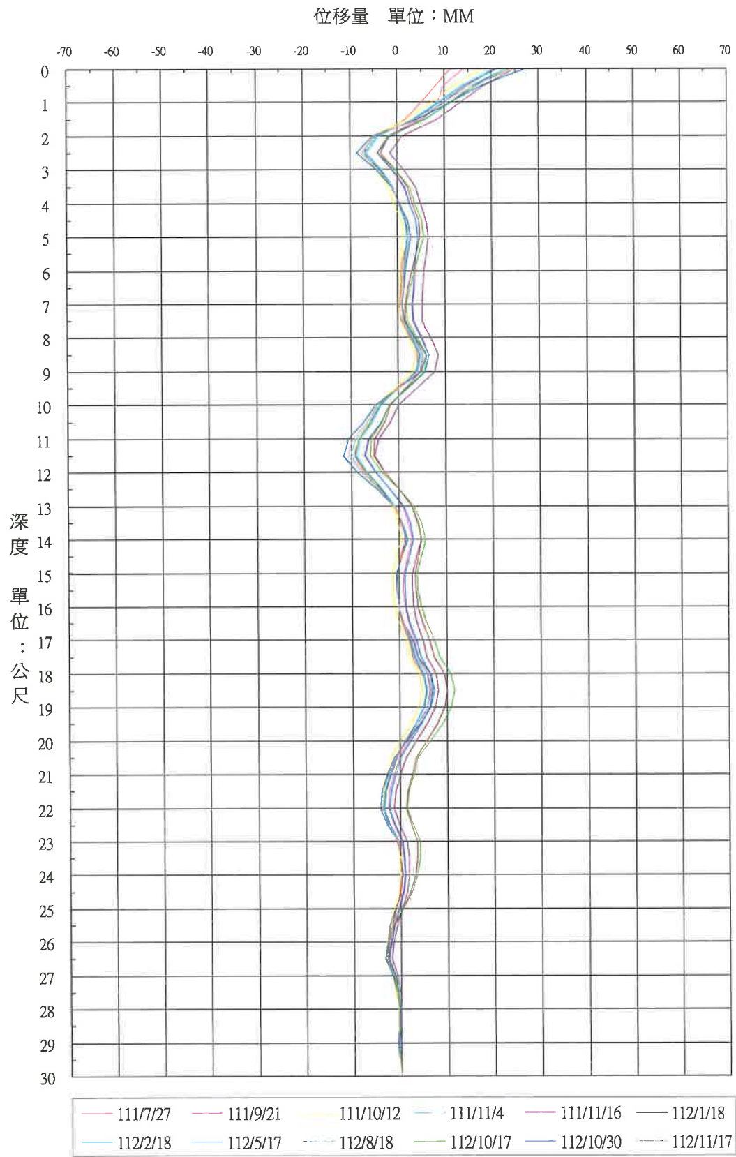
圖2.4-1 傾斜管測量位移量曲線圖(SI1-A)
