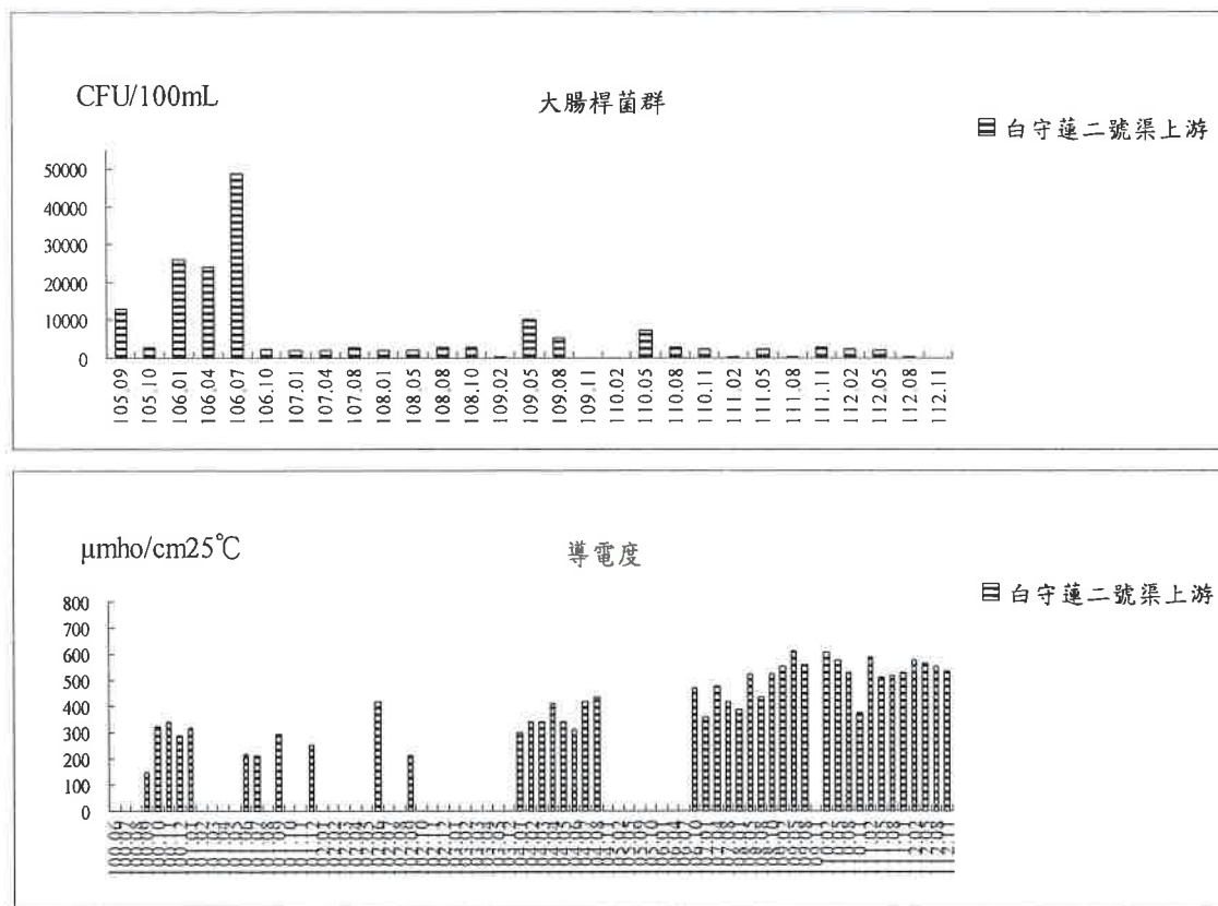
圖 3.5-1 白守蓮二號渠上游地面水水質監測結果趨勢圖(續二)
