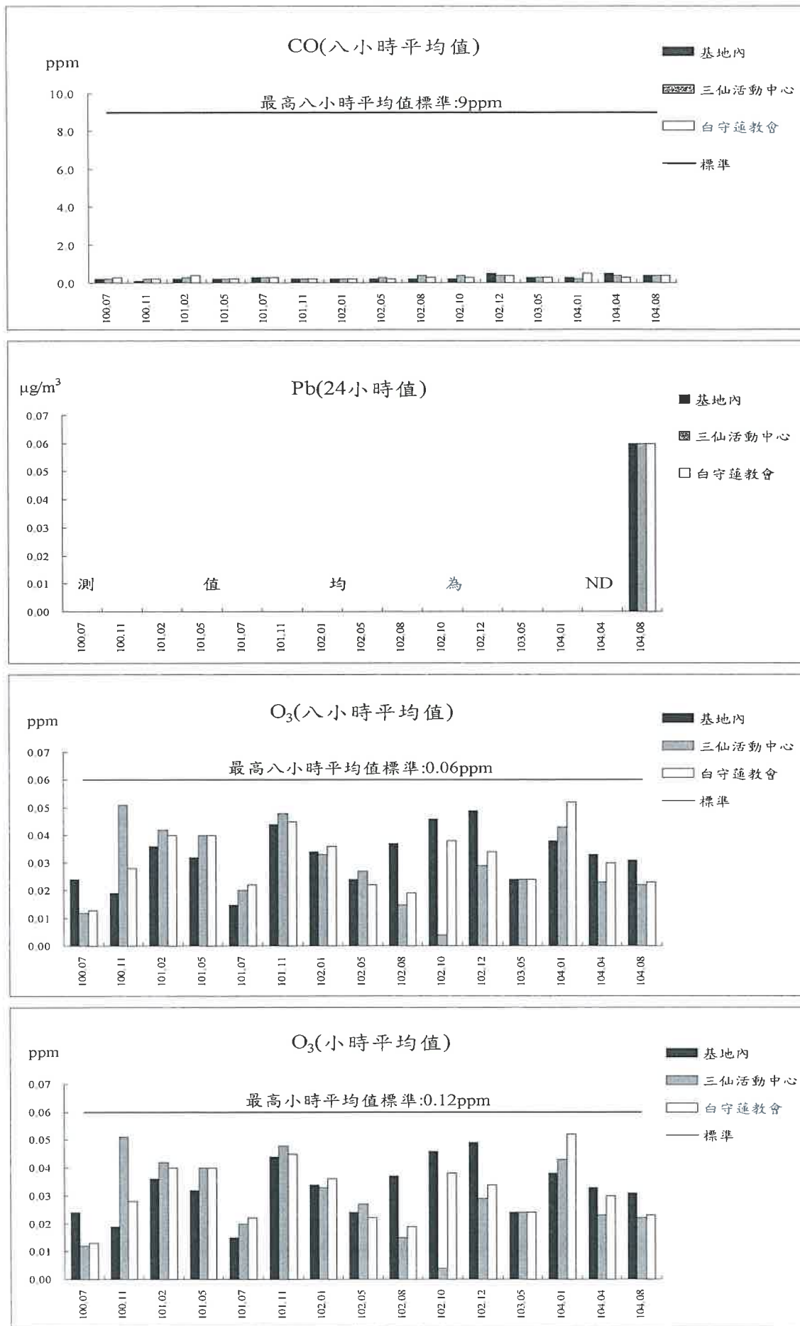
圖3.1-1 歷次空氣品質測值變化圖(續二)
