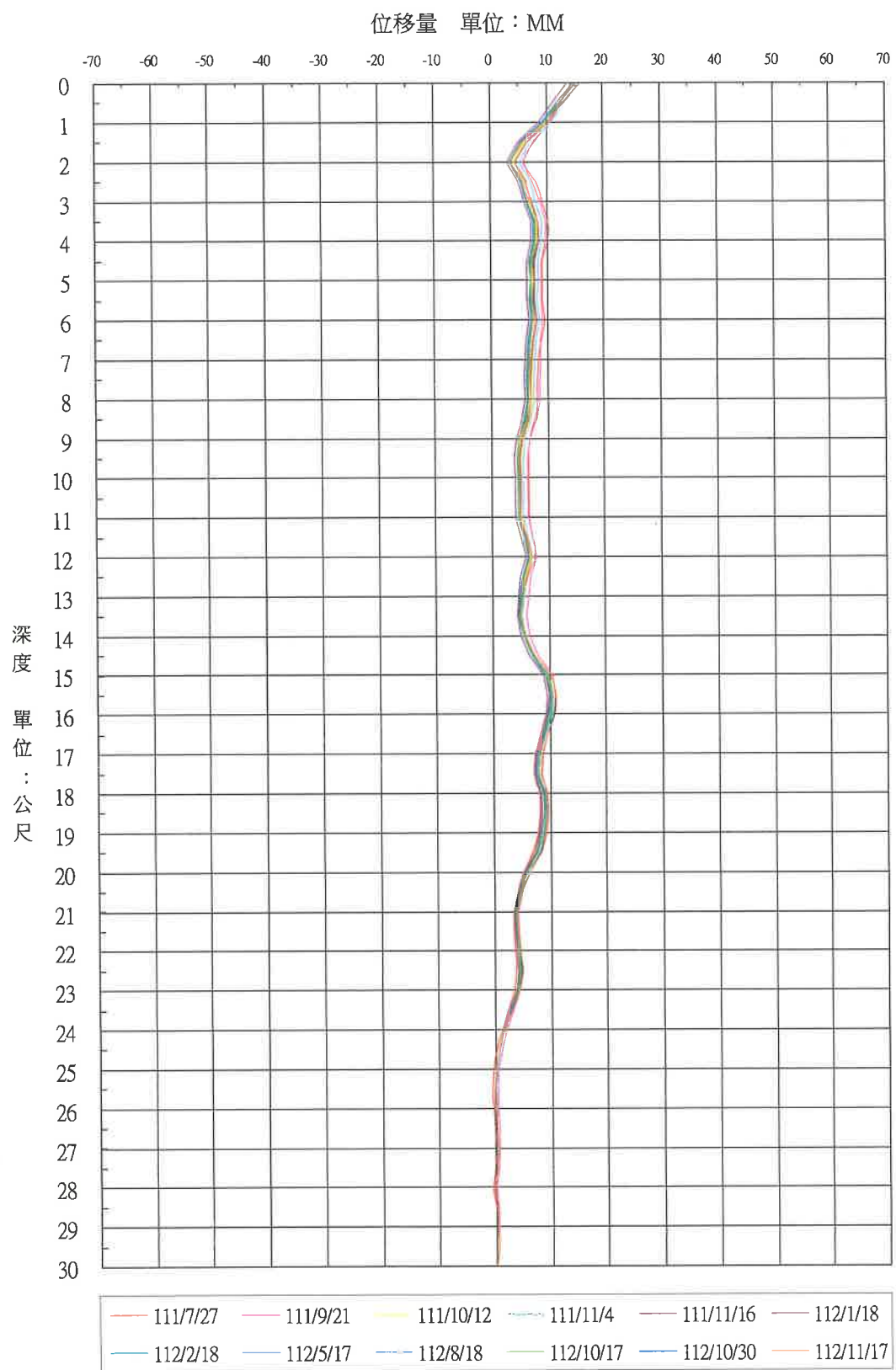
圖2.4-2 傾斜管測量位量曲線圖(SI1-B)
