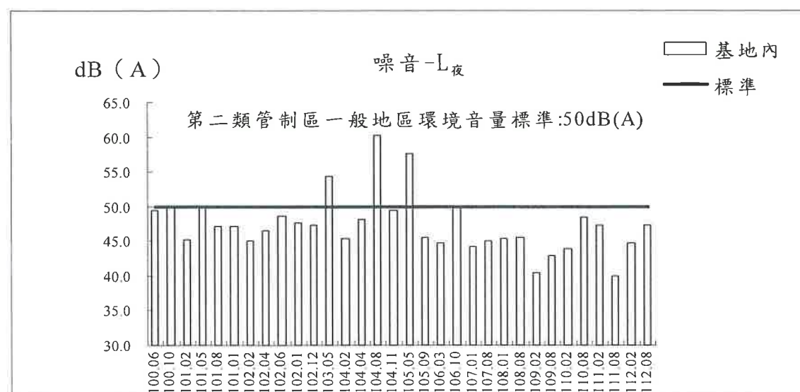
圖3.2-1 基地內測站歷次噪音測值變化圖
