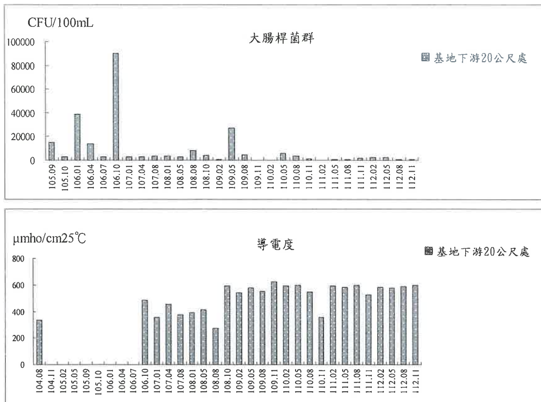
圖 3.5-2 基地下游 20 公尺處地面水水質監測結果趨勢圖(續二)
