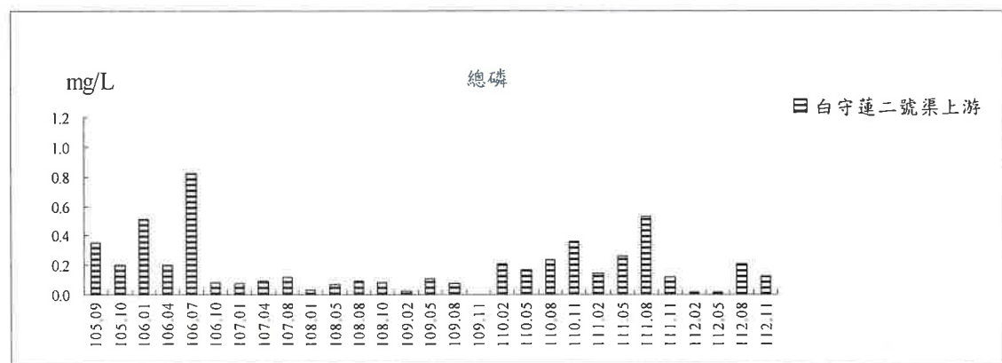
圖 3.5-1 白守蓮二號渠上游地面水水質監測結果趨勢圖(續一)
