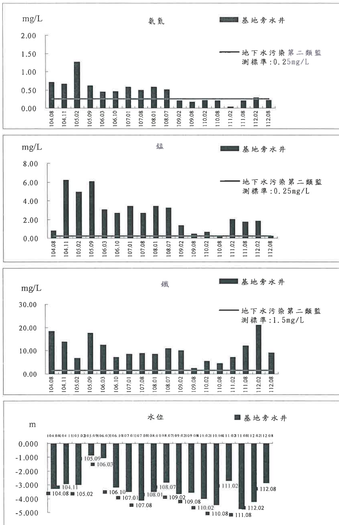
圖 3.7-1 地下水水質監測結果趨勢圖
