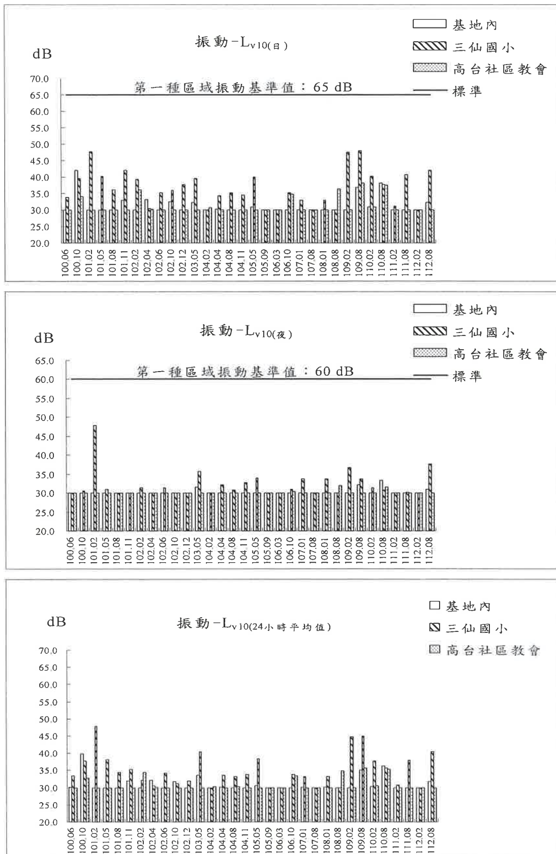
圖3.3-1 歷次振動測值變化圖
