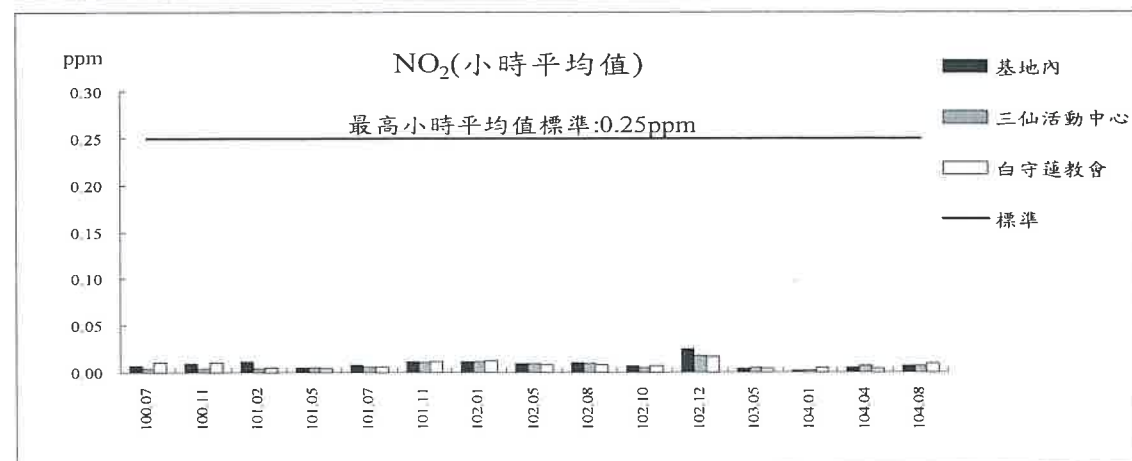
圖 3.1-1 歷次空氣品質測值變化圖
