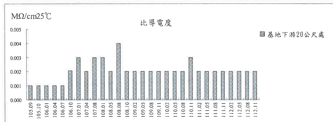
圖 3.5-2 基地下游 20 公尺處地面水水質監測結果趨勢圖
