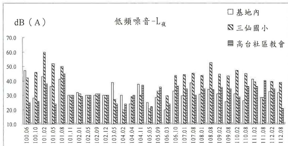
圖3.4-1 歷次低頻噪音測值變化圖
