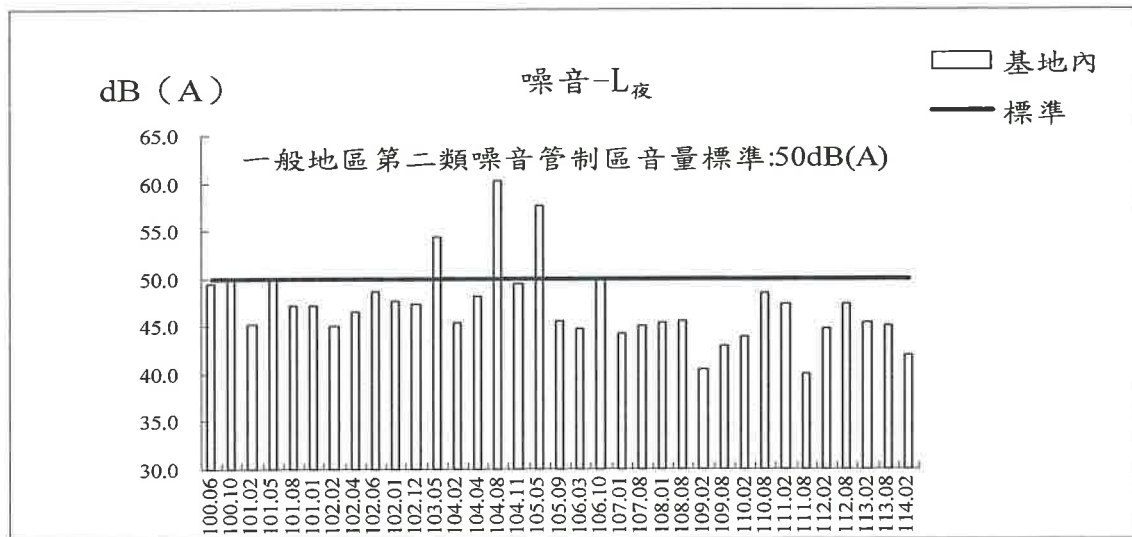
圖3.2-1 基地內測站歷次噪音測值變化圖
