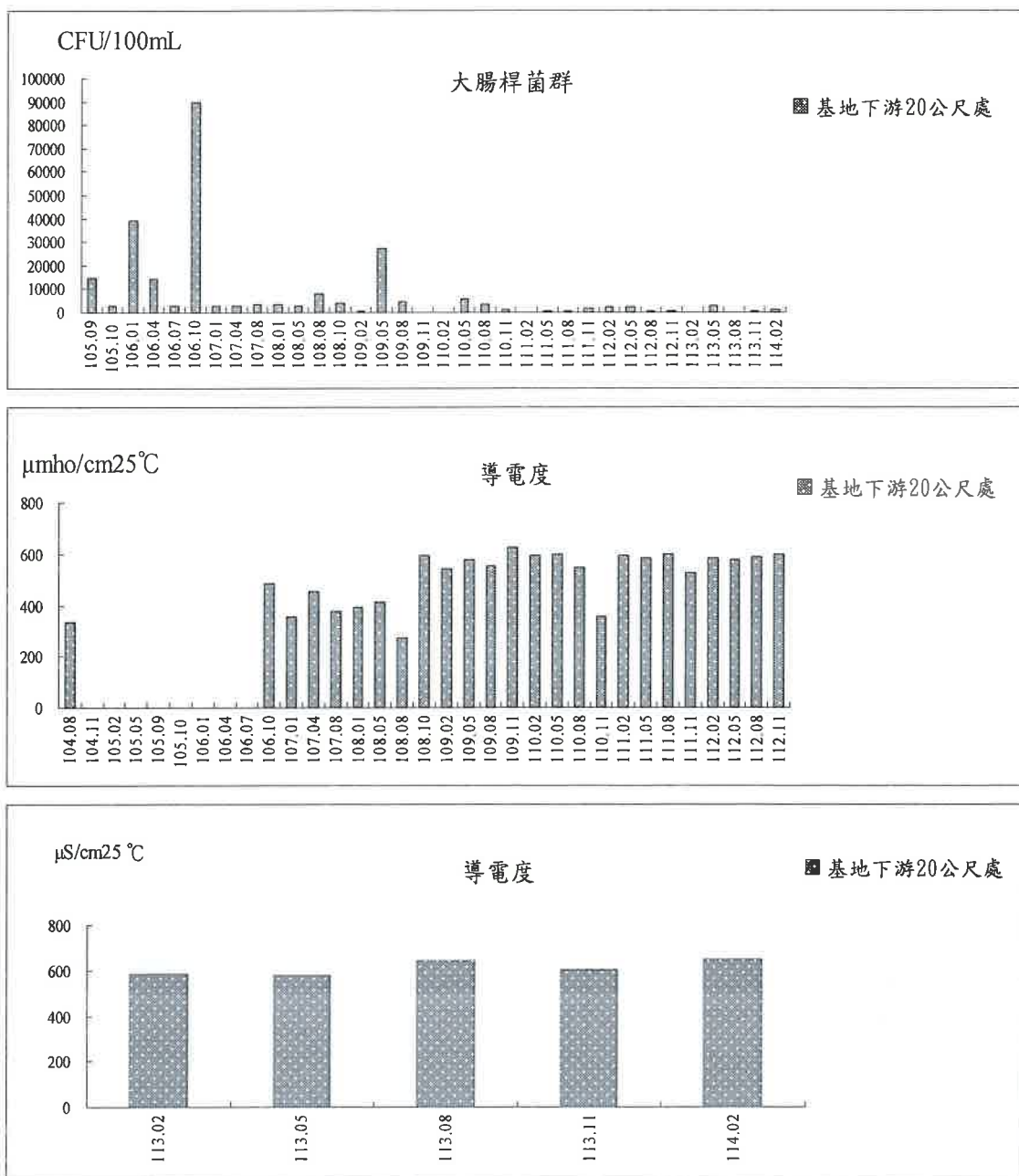
圖 3.5-2 基地下游 20 公尺處地面水水質監測結果趨勢圖(續二)
