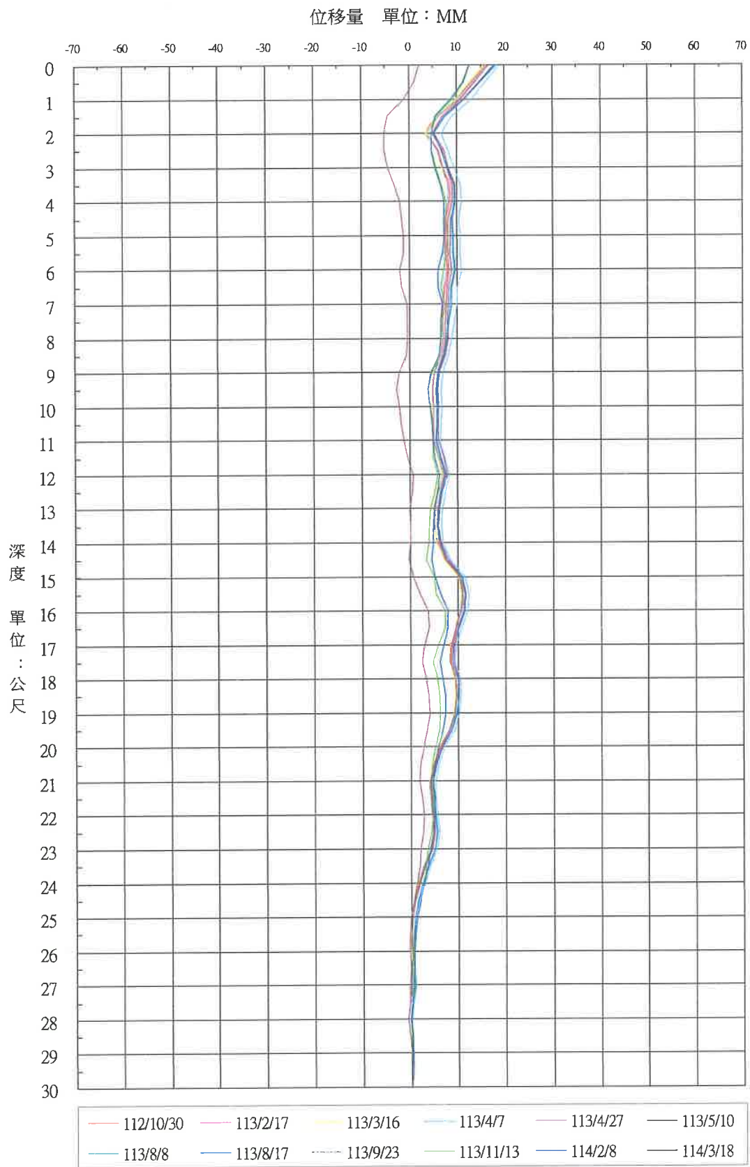
圖2.8-2 傾斜管測量位移量曲線圖(SI1-B)
