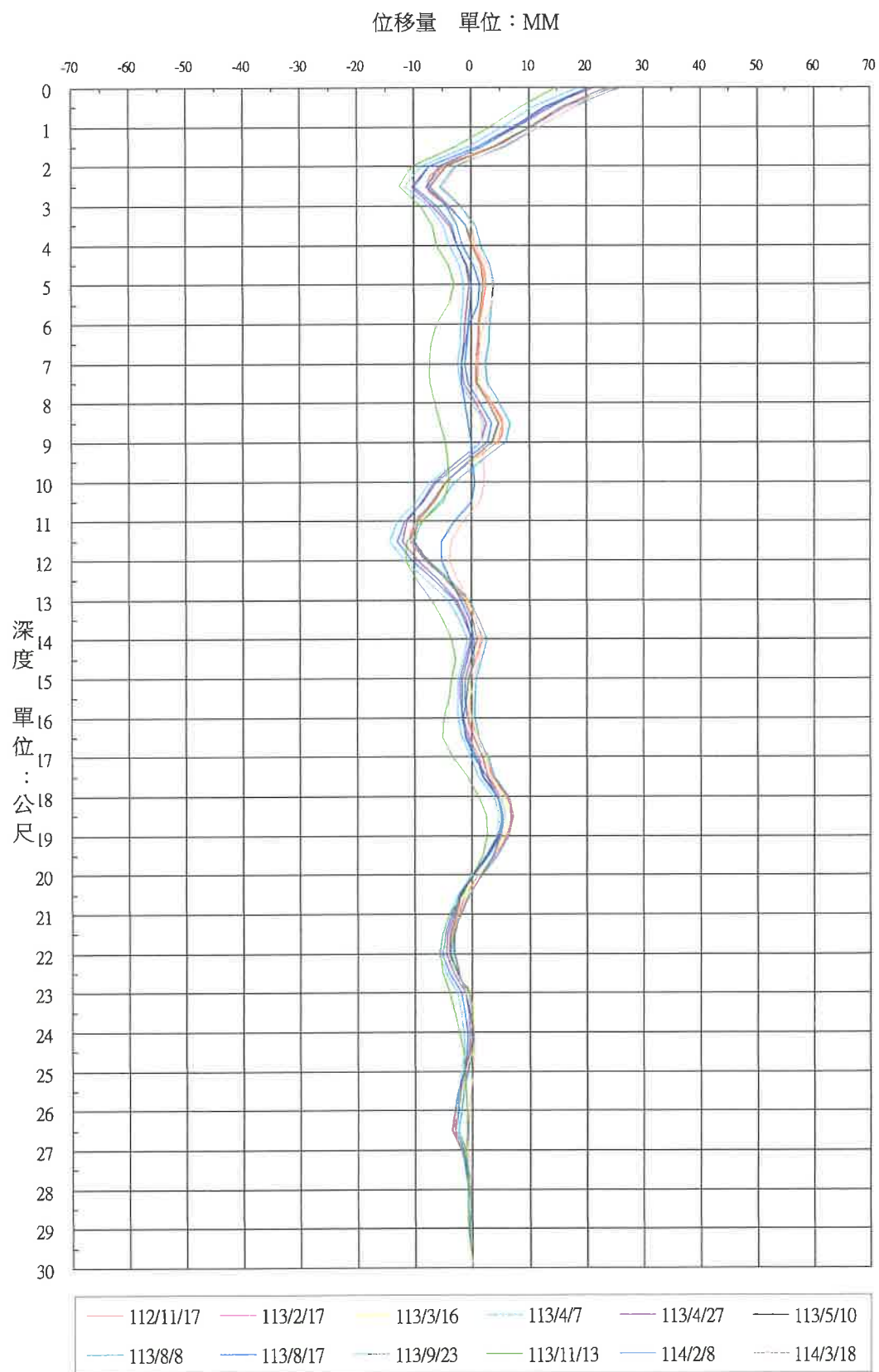
圖2.8-1 傾斜管測量位移量曲線圖(SI1-A)
