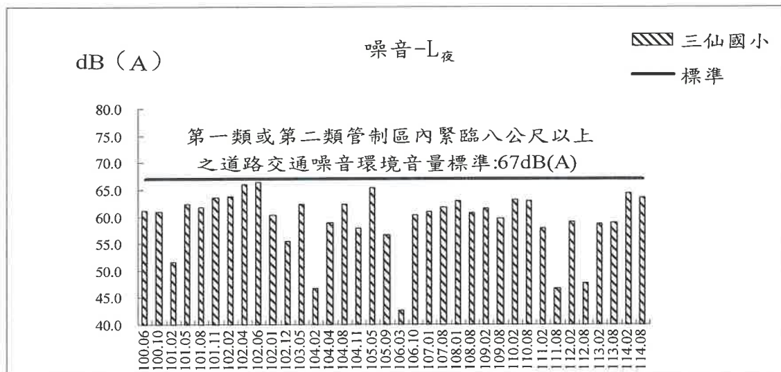
圖3.2-2 三仙國小測站歷次噪音測值變化圖
