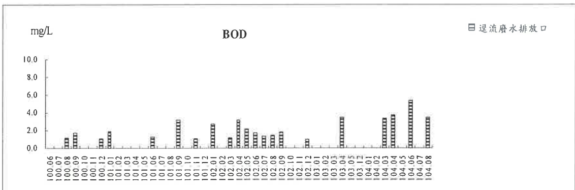
圖 3.5-3 逕流廢水排放口地面水水質監測結果趨勢圖
