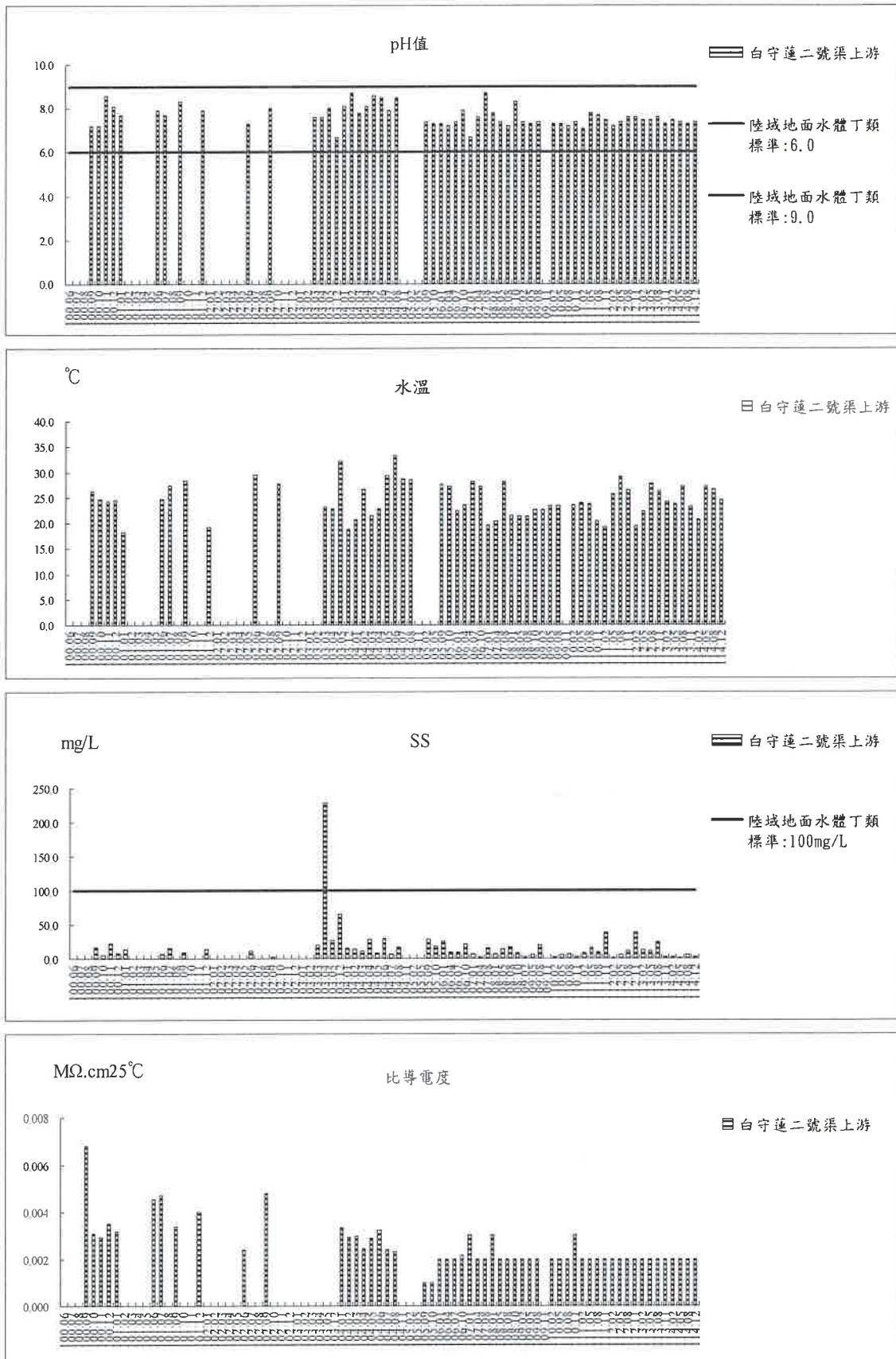
圖 3.5-1 白守蓮二號渠上游地面水水質監測結果趨勢圖
