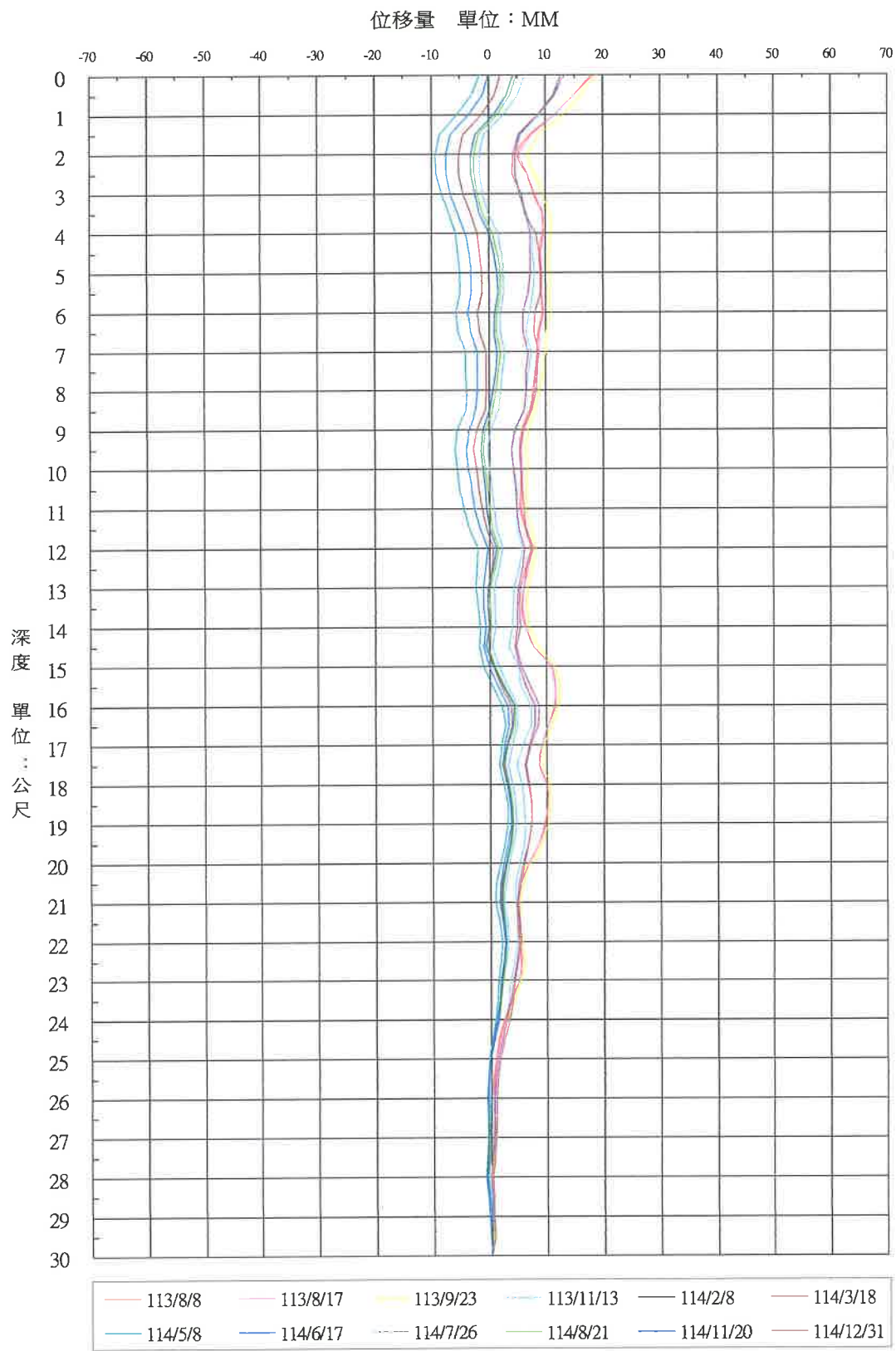
圖2.4-2 傾斜管測量位移量曲線圖(SI1-B)
