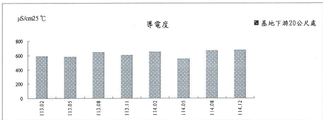
圖 3.5-2 基地下游 20 公尺處地面水水質監測結果趨勢圖(續二)
