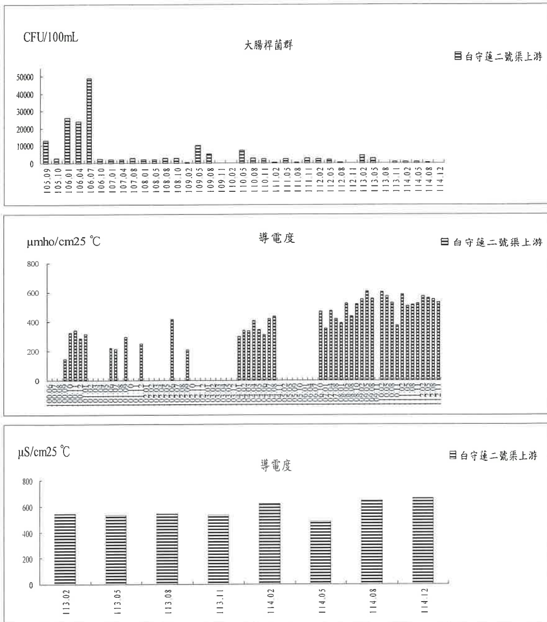
圖 3.5-1 白守蓮二號渠上游地面水水質監測結果趨勢圖(續二)
