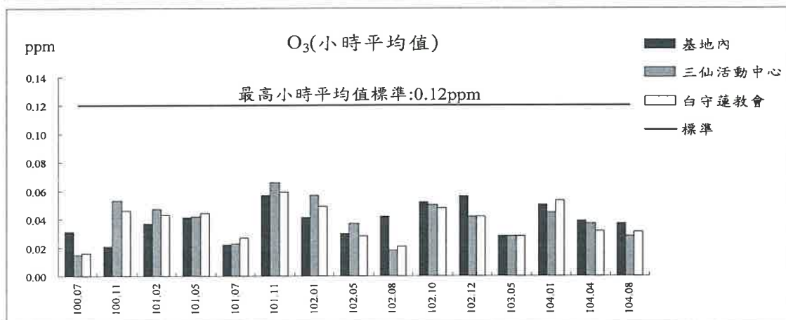
圖3.1-1 歷次空氣品質測值變化圖(續二)
