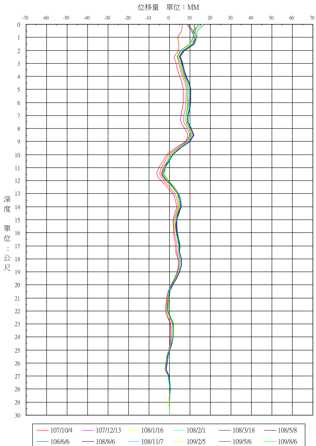
圖2.8-1 傾斜管測量位移量曲線圖(SI1-A)
