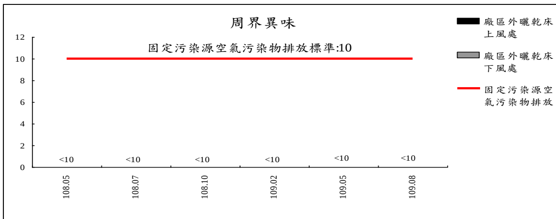
圖3.1-2 歷次周界異味測值變化圖
