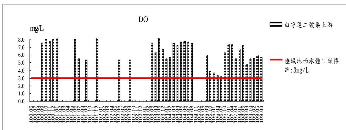
圖 3.5-1 白守蓮二號渠上游地面水水質監測結果趨勢圖
