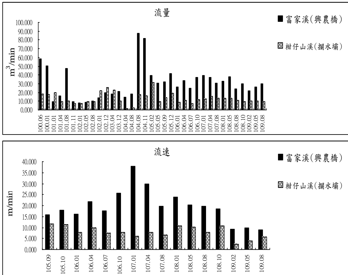
圖 3.6.1 地面水水文監測結果趨勢圖
