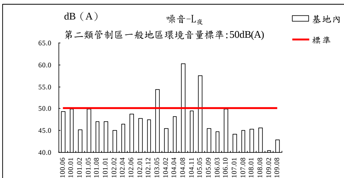
圖3.2-1 基地內測站歷次噪音測值變化圖
