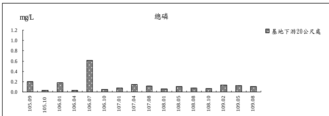
圖 3.5-2 基地下游 20 公尺處地面水水質監測結果趨勢圖(續一)
