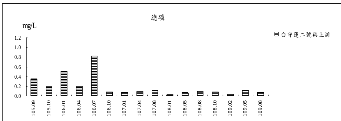
圖 3.5-1 白守蓮二號渠上游地面水水質監測結果趨勢圖(續一)
