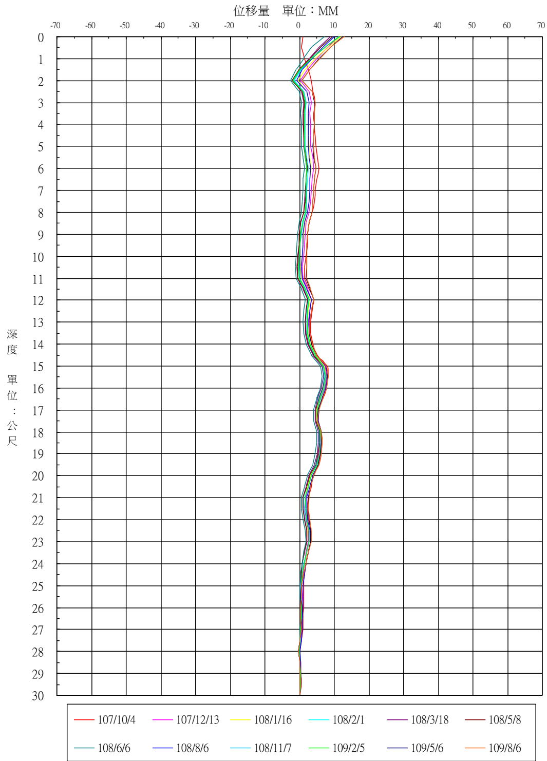
圖2.8-2 傾斜管測量位置曲線圖(SI1-B)
