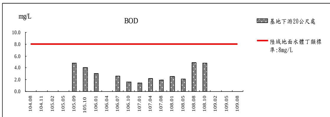
圖 3.5-2 基地下游 20 公尺處地面水水質監測結果趨勢圖
