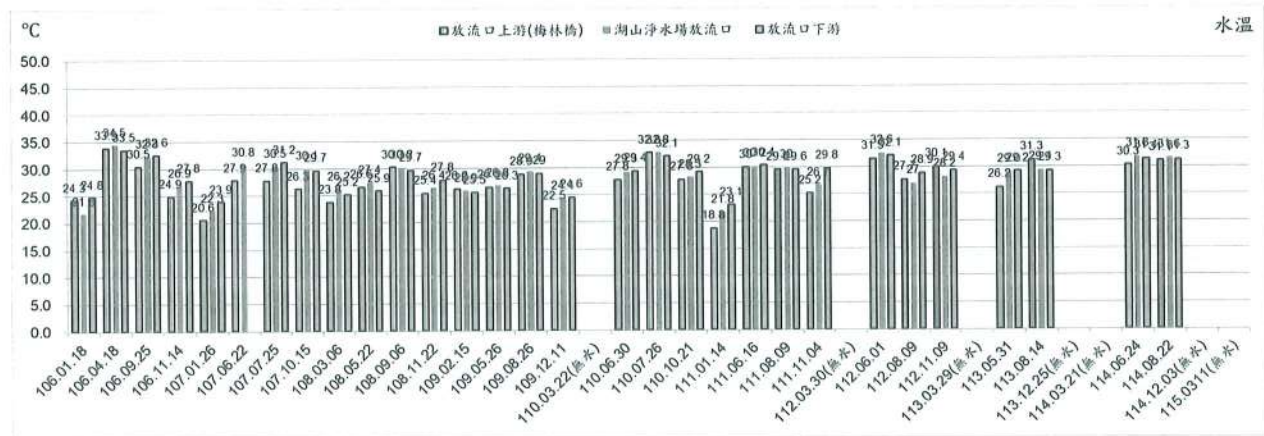
圖 2.3- 2、河川水質歷次監測結果彙整圖(水溫)
