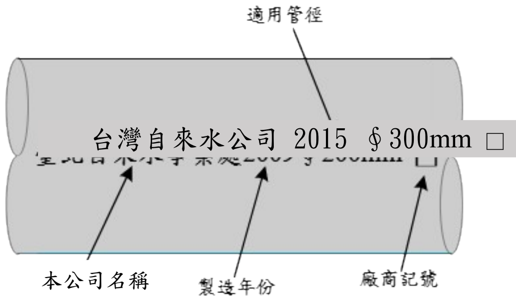
直管用 PE 套膜標示參考圖
