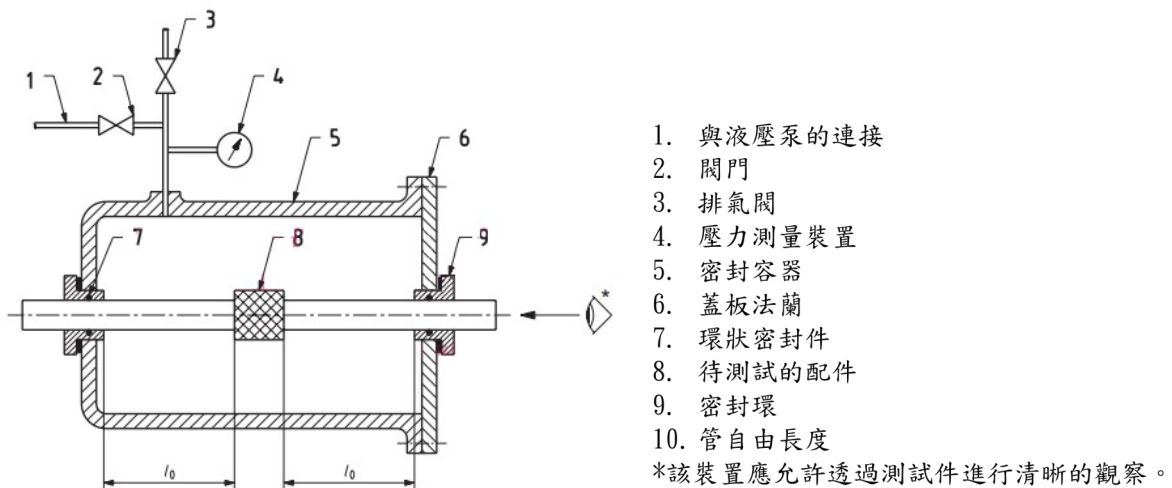
圖 7 負壓試驗裝置例(僅適用於管徑 \leq 63\text{mm} )
