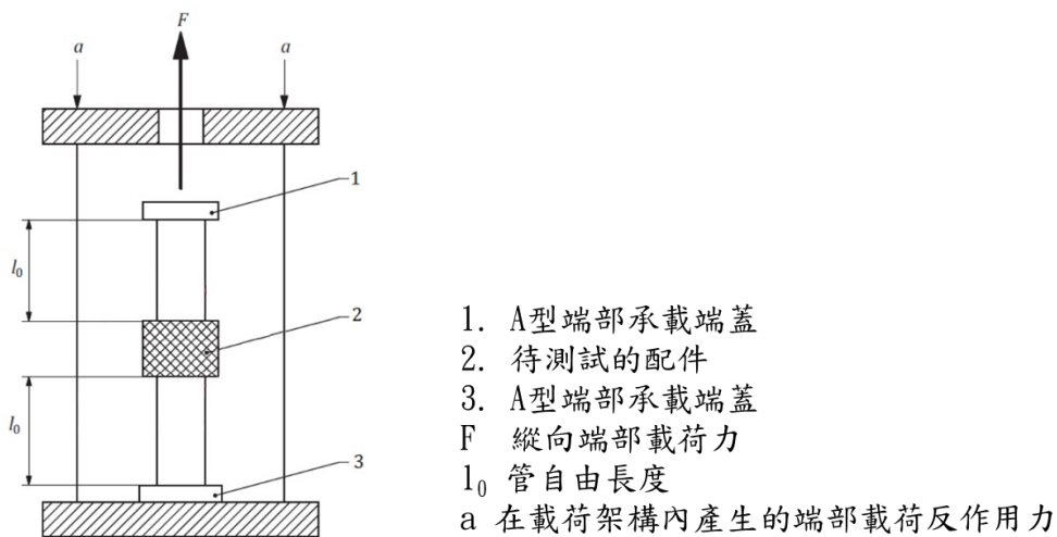
圖 5 抗拉試驗裝置例
