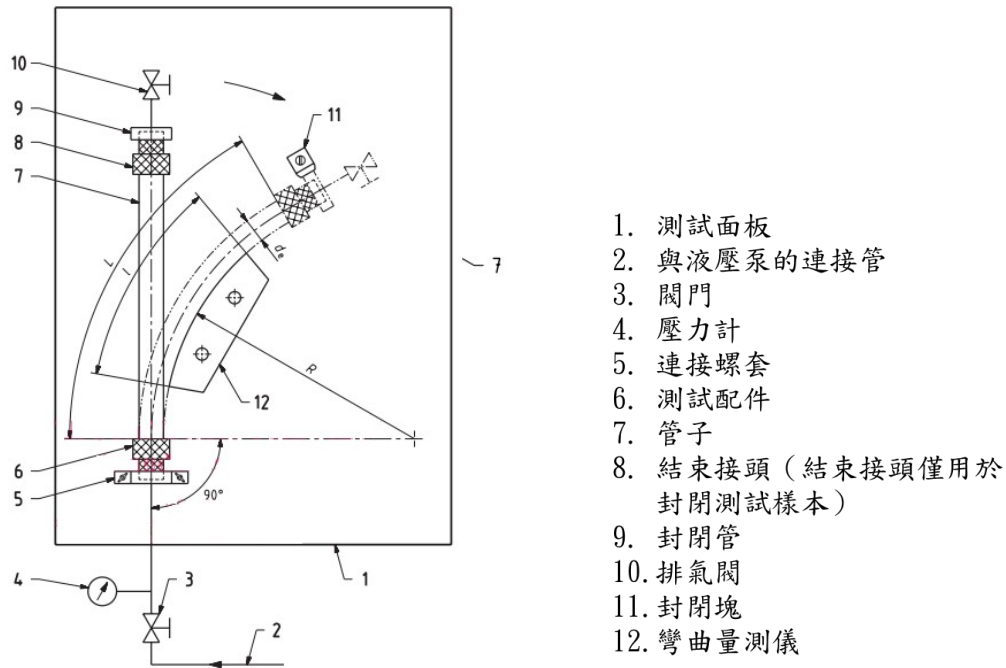
圖 6 承受彎曲時的內壓密封性試驗裝置例
