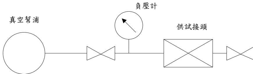
圖 3 負壓試驗裝置例
