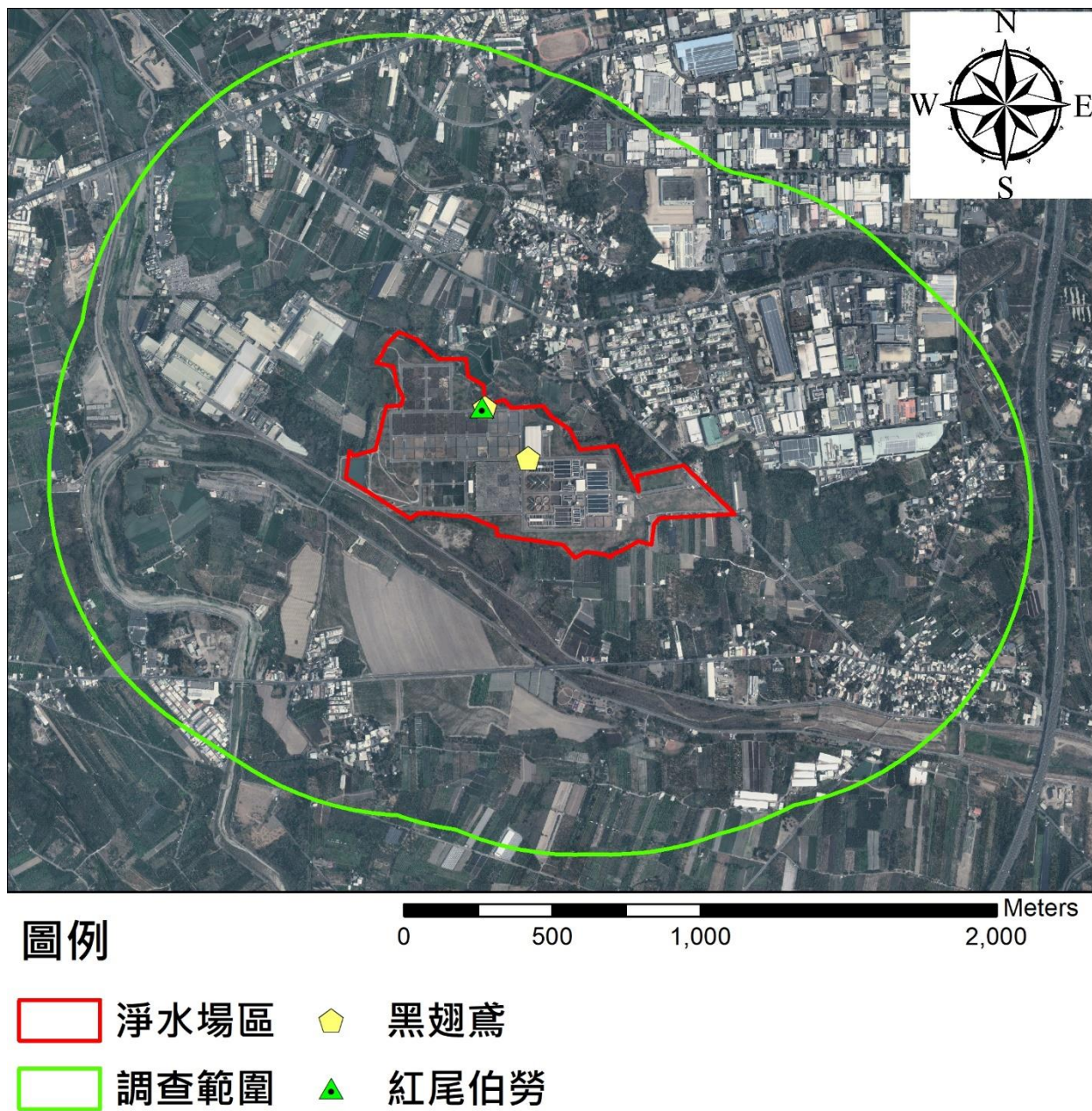
圖 2.5- 4、湖山淨水場本季保育類動物分布圖
