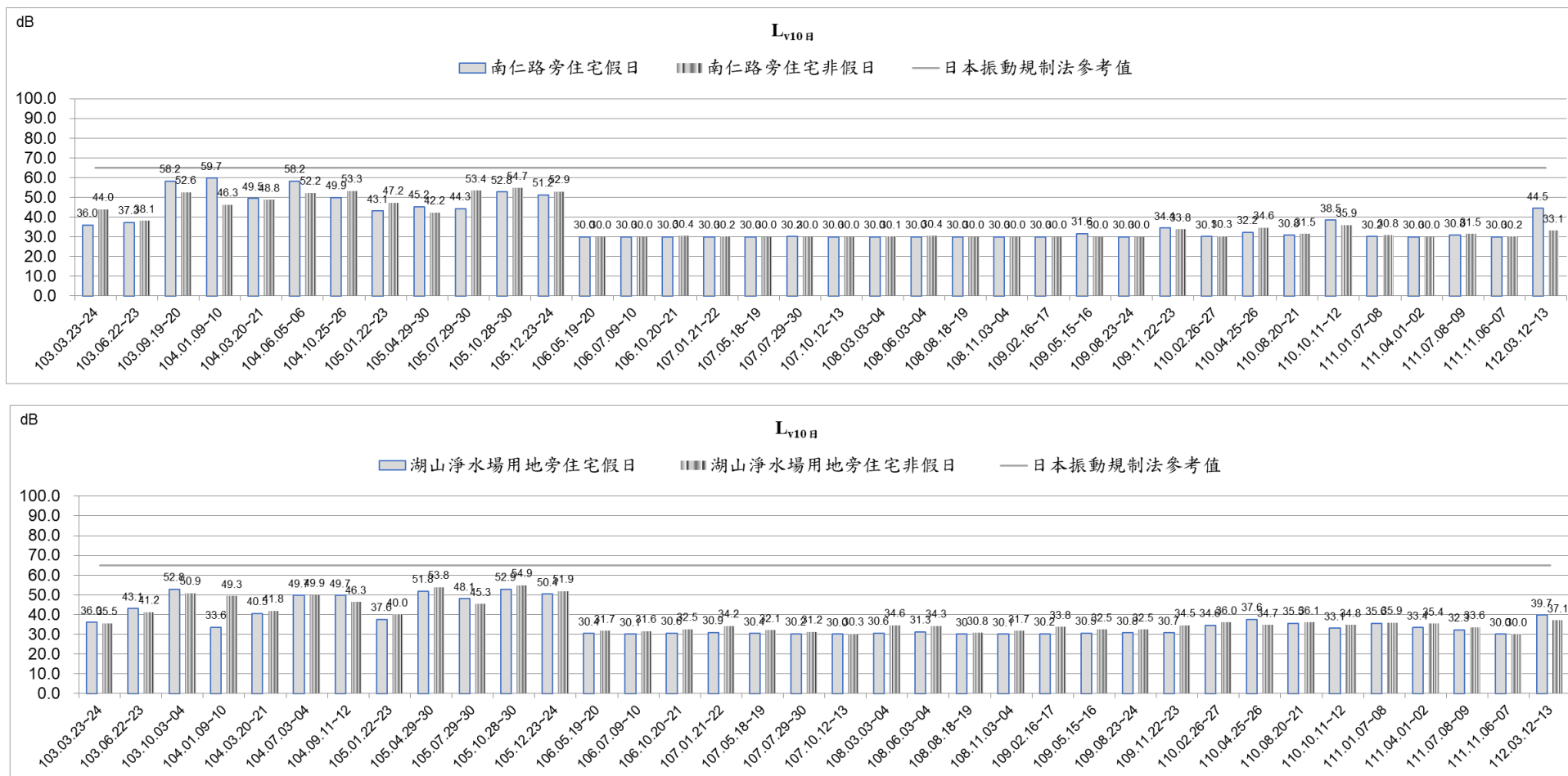
圖 2.1- 4、振動監測結果彙整圖(L v10 日)
