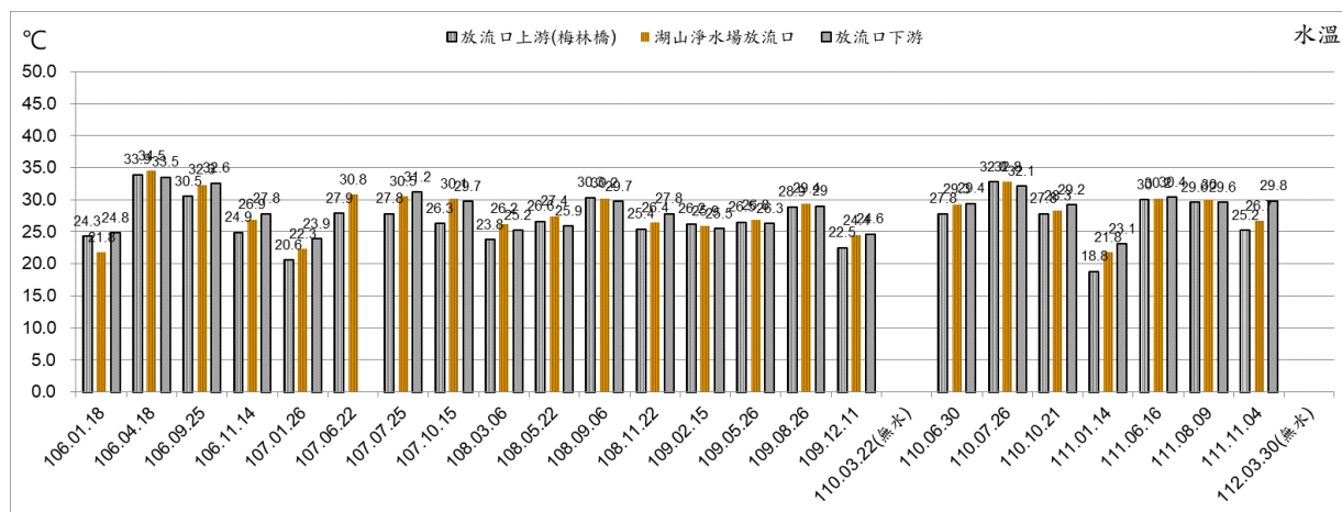
圖 2.3- 2、河川水質歷次監測結果彙整圖(水溫)
