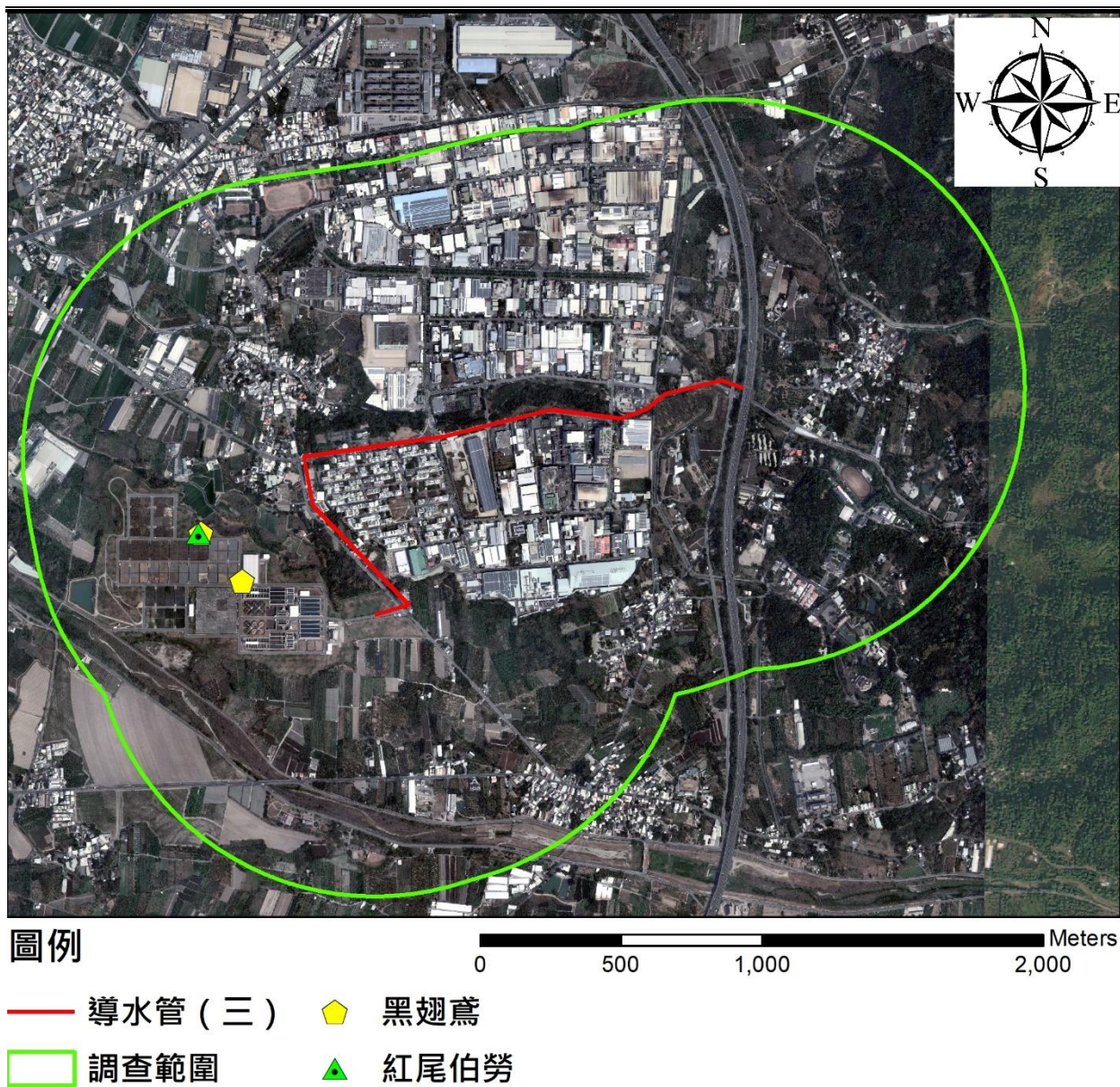
圖 2.5- 10、導水管 (三) 本季保育類動物分布圖
