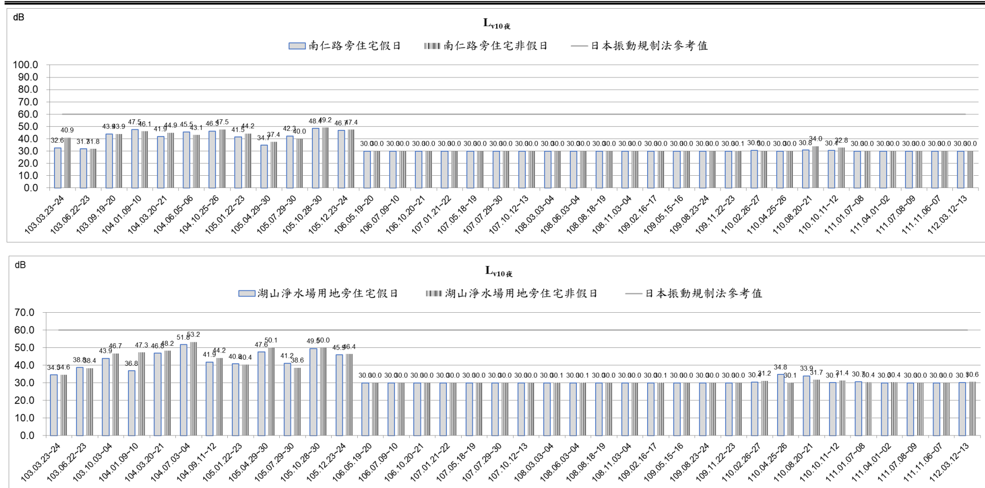
圖 2.1- 5、振動監測結果彙整圖( L_{v10} 夜)
