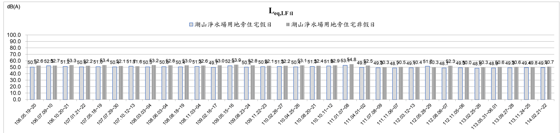
圖 2.2- 1、低頻噪音監測結果彙整圖( L_{eq,LF 日} )
