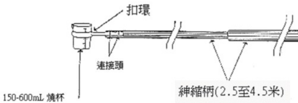
(圖一)採樣杓
