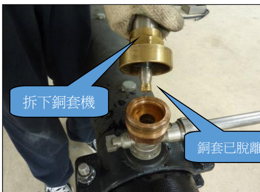
(鬆開轉接頭拆下銅套機)
