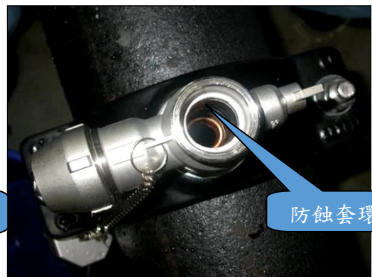
(防蝕套環裝置完成)
