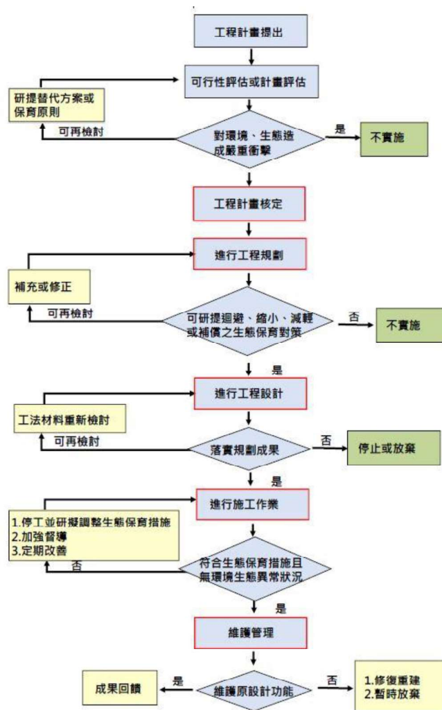
圖二、公共工程生態檢核作業流程
