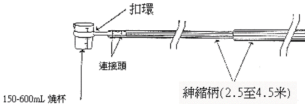
(圖一)採樣杓
