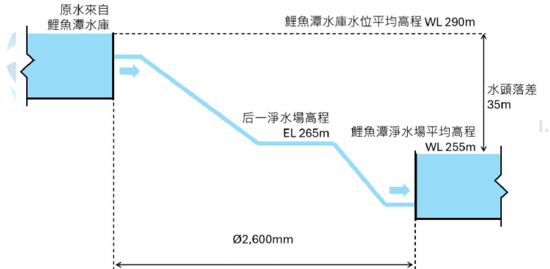
圖三、水頭條件 - 縱斷面示意圖
